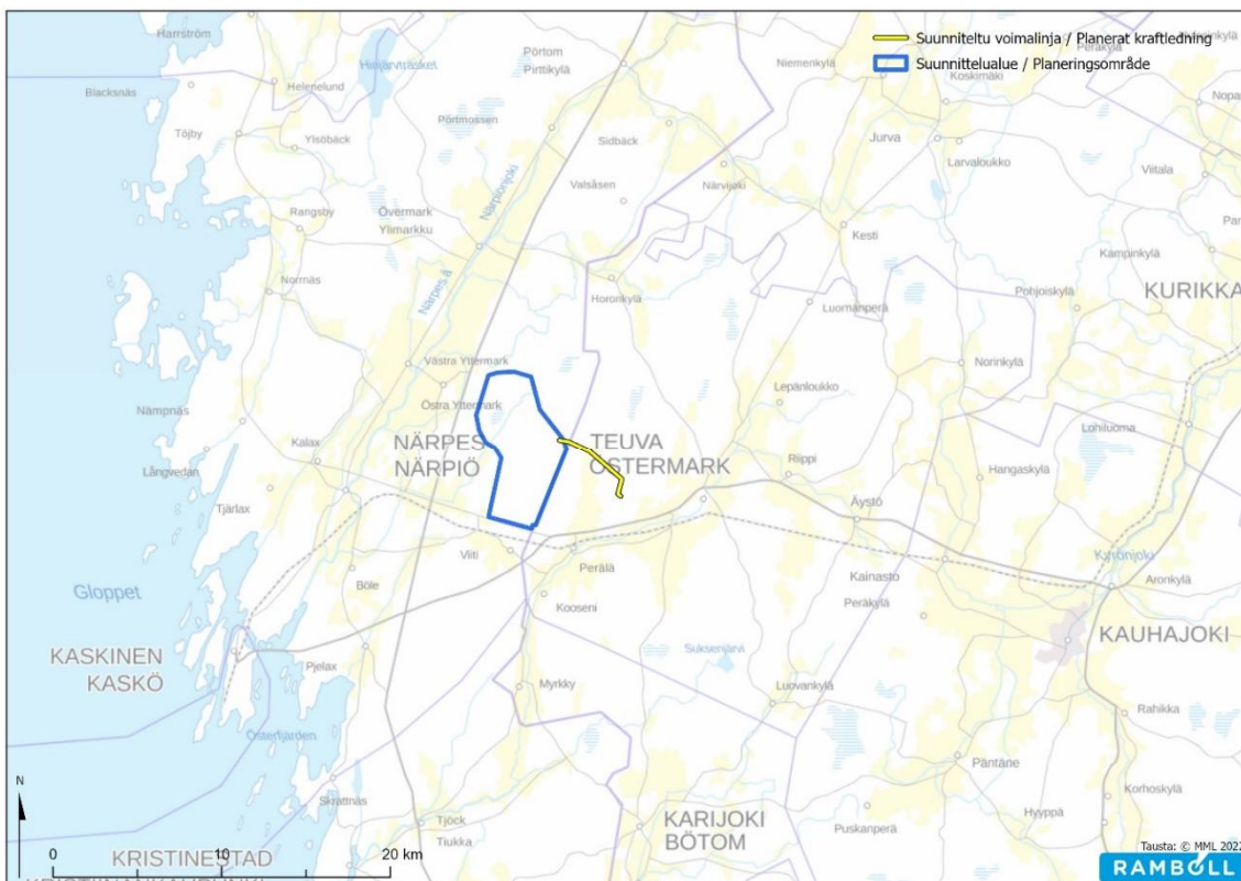
Bild 1. Vindkraftsparkens läge.
